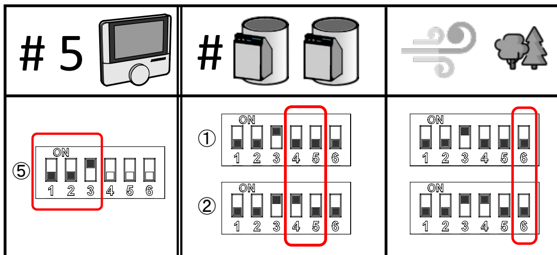
Obrázek 25 – Příklad přívodu: Zóna pět, dvě klapky, přívod.
