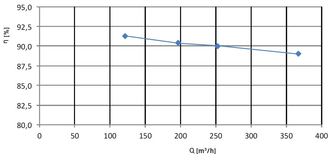
Obrázek 7 – Účinnost rekuperace
