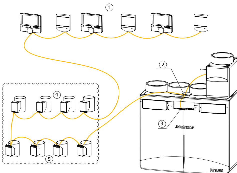
Obrázek 10 – Topologie připojení
