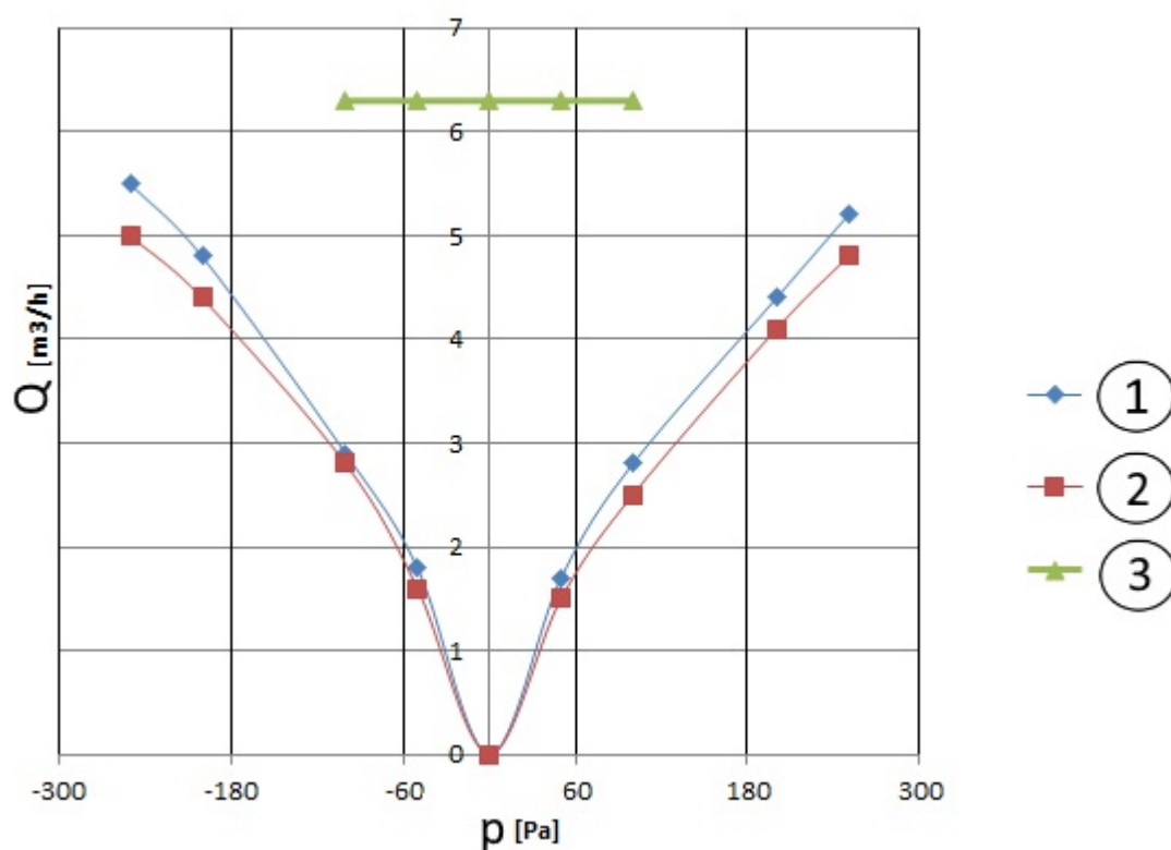
Obrázek 6 – Netěšnost
