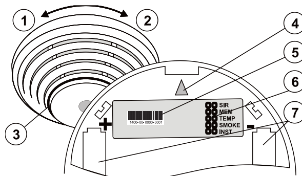
Obrázek 1: 1 – otevření detektoru; 2 – zavření detektoru; 3 – optická signalizace stavu; 4 – orientační šipka pro nasazení; 5 – sériové číslo; 6 – konfigurační propojky; 7 – prostor pro vložení baterií
