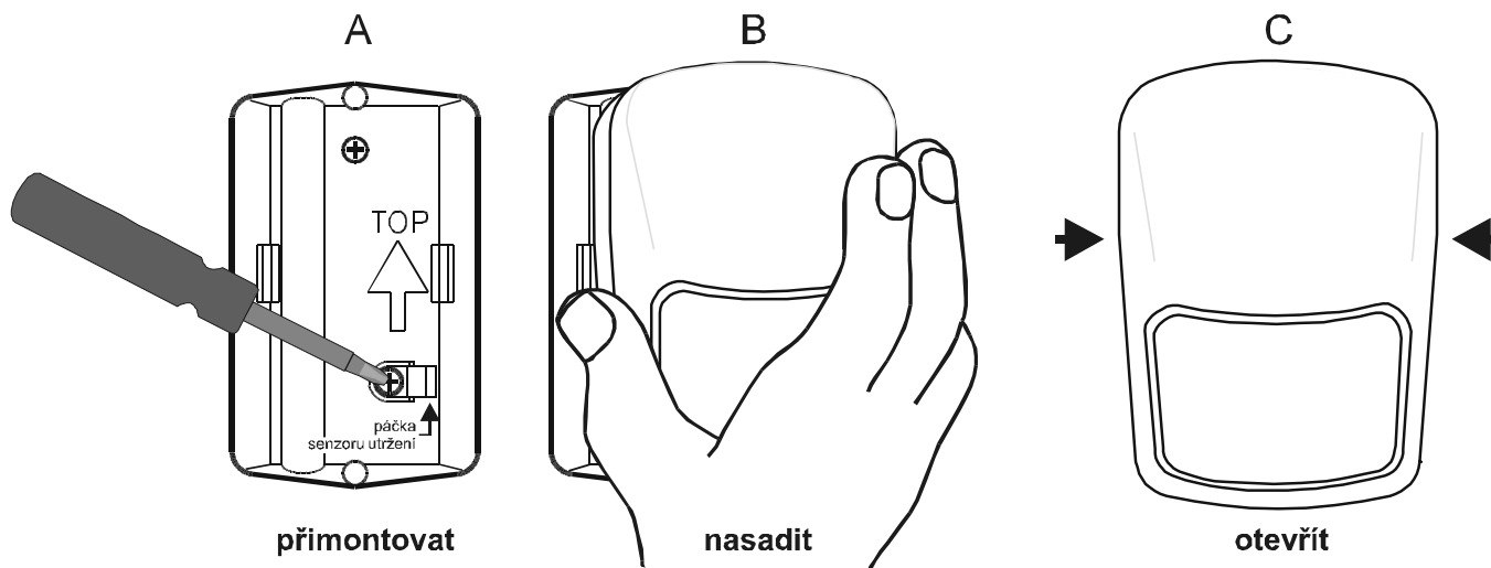
Obr.9 – montáž detektoru pohybu
