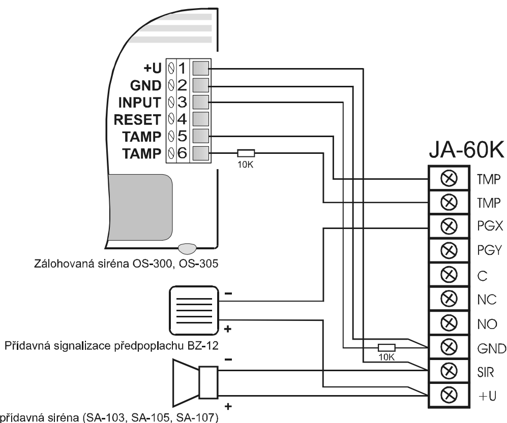
Obr.14 – příklad zapojení „drátových“ periférií k ústředně JA-60K
