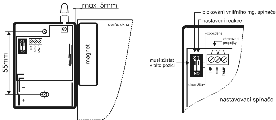
Obr.8 – montáž detektoru dveří a nastavení reakce
