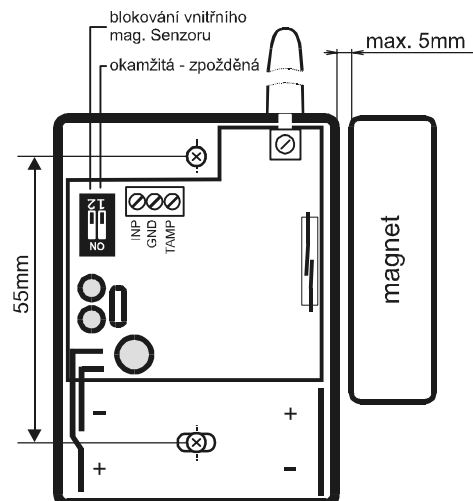
Obr.15 – magnetický detektor
