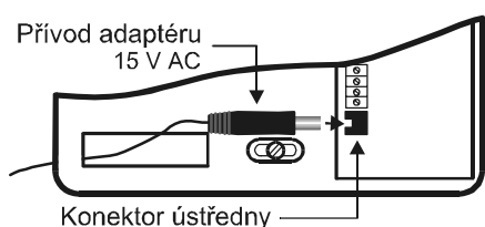
Obr.3 – zapojení adaptéru
