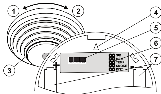
Abbildung 3: 1 - Melder öffnen; 2 - Melder schließen; 3 - optische Statusanzeige; 4 - Pfeil zeigt an, wo der Melder eingehängt werden soll; 5 - Seriennummer; 6 - Drahtbrücken; 7 - Batterieeinfachung
