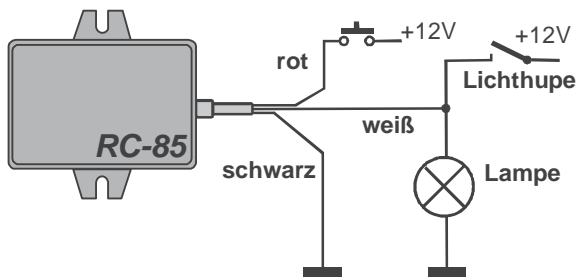
Beispiel einer Verdrahtung in einem Fahrzeug
