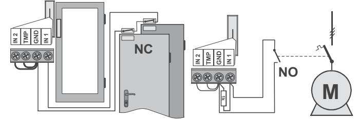
Beispiel des Anschließens der externen Sensoren mit dem Öffnungs- und Schließkontakt
