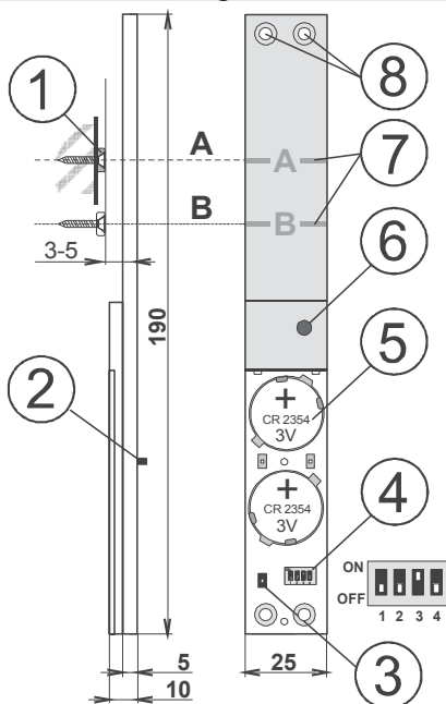
1. Magnet; 2. Hintere Sabotagekontakte; 3. Sabotagekontakt im Gehäuse; 4. DIP-Schalter; 5. Batterie; 6. LED- Meldeleuchte; 7. Markierungen für die Detektion; 8. Montageöffnungen
