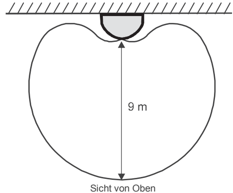
Erfassungsbereich des Glasbruchsensoren
