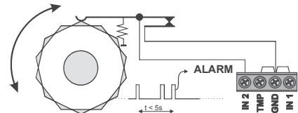
Beispiel des Anschließens des Eingangs IN2
