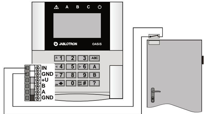
Abb. 2 Anschluss des Türöffnungsmelders
