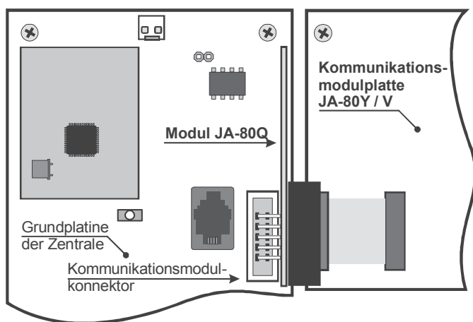
Abb. 1 Modulschaltung
