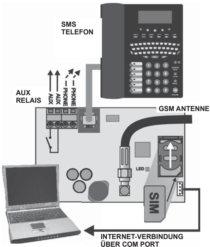
Abb. 1 Verdrahtung des Kommunikationsmoduls
