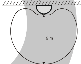
Detekčné pokrytie detektora – pohľad zhora i zboku
