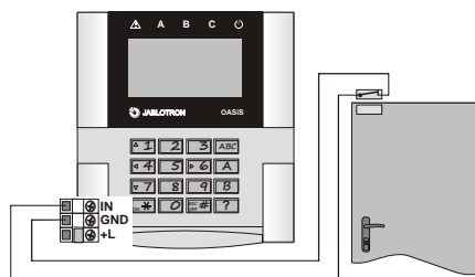
Príklad zapojenia detektora otvorenia dverí
