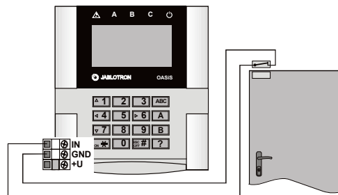
Příklad připojení dveřních detektorů
