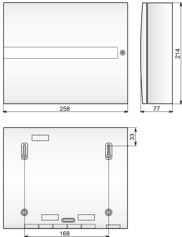
obr. 2 Rozměry skříňě opakovače
