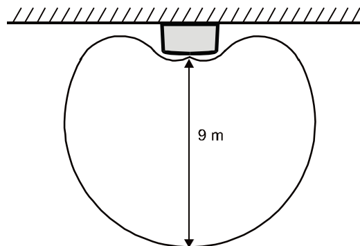
Záběrová charakteristika detektoru rozbití skla
