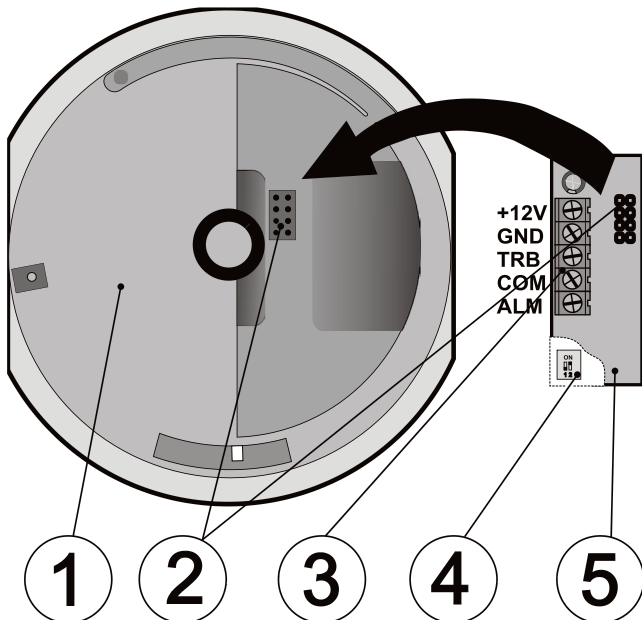
Obrázek: 1 – Detektor Ei208(D)W, 2 – systémový konektor pro propojení s Ei208(D)W, 3 – svorkovnice, 4 – přepínače DIP pro volbu funkce výstupů (na spodní straně modulu), 5 – drátový modul GS-208-CO
