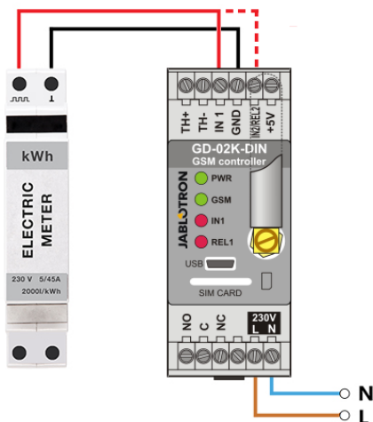
Figur 6: Strømforbruksmålingsmodus.
