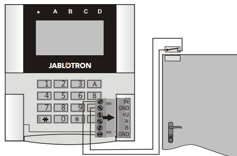
Obr. 2: Pripojenie detektora otvorenia dverí
