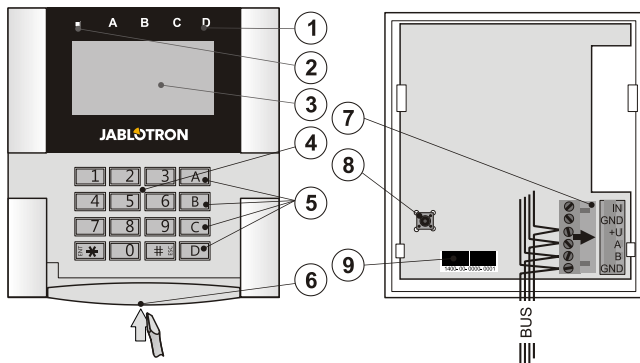
Obr.1: 1 – stavové indikátory A, B, C, D; 2 – systémový indikátor; 3 – LCD displej; 4 – klávesnica s RFID čítačkou; 5 – funkčné tlačidlá A, B, C, D; 6 – západka pre otvorenie klávesnice; 7 – odnímateľná svorkovnica zbernice so svorkami pre pripojenie detektora; 8 – sabotážny kontakt; 9 – sériové číslo.
