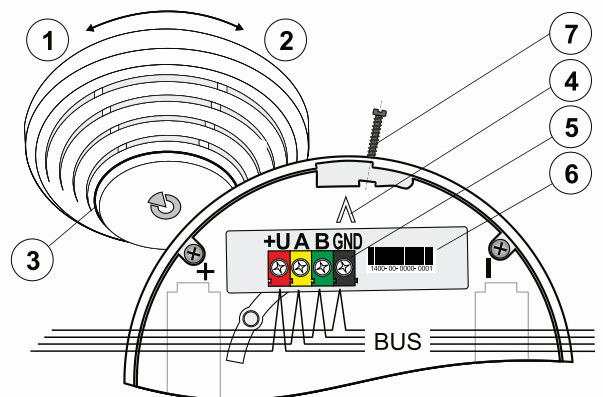
obrázek 6: 1 – uvolnění (sejmutí) detektoru; 2 – upevnění (nasazení) detektoru; 3 – optická signalizace; 4 – orientační šipka pro nasazení; 5 – svorky sběrnice; 6 – sériové číslo; 7 – aretační šroub
