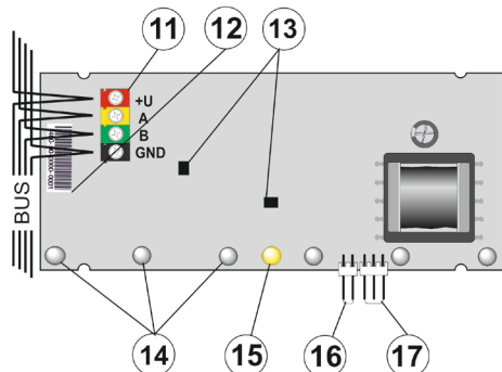
Obrázek: 11 – svorky sběrnice; 12 – sériové číslo; 13 – sabotážní senzory; 14 – vysoce svítivé signální blikače; 15 – systémová žlutá signálka; 16 – připojení akumulátoru; 17 – připojení elektroakustického měniče (pozor vysoké napětí)
