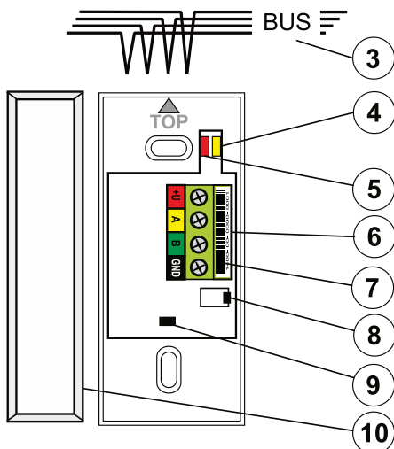
obrázek: 3 – kabel sběrnice; 4 – žlutá signálka porucha; 5 – červená signálka aktivace; 6 – svorky sběrnice; 7 – sériové číslo; 8 – sabotážní spínač; 9 – magnetický snímač; 10 – magnet
