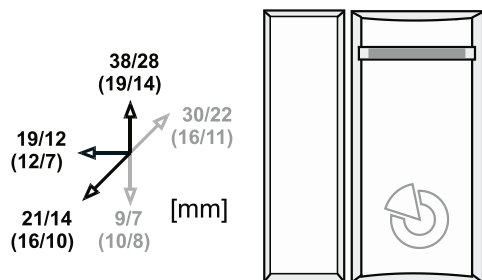
obrázek: orientační detekční vzdálenost – aktivace/deaktivace na nemagnetickém (magnetickém) povrchu
