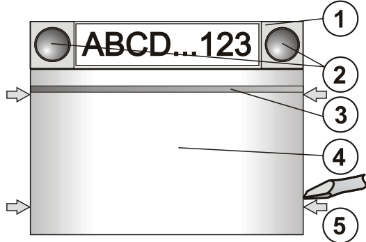
Figur: 1 – funktion segment; 2 - funktion knapper; 3 - baggrundsbelyst aktiveringsknop; 4 – RFID modul; 5 – pal til åbning af enheden
