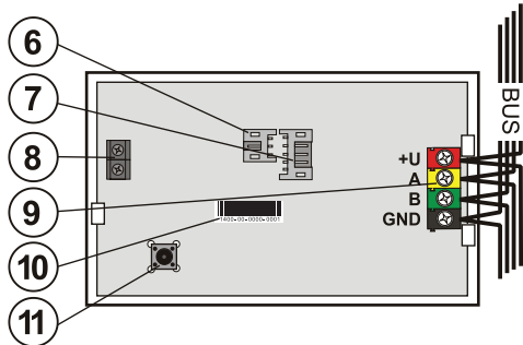
Figur: 6 – lyd moduls stik; 7 – statussegments stik; 8 - terminal for tilslutning af lyd modulet til centralen, 9 – BUS terminaler, 10 - produktkode 11 - sabotagekontakt
