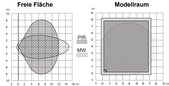
Abb. 3: Erfassungseigenschaften bei freier Fläche und in einem Modellraum – Installation in einer Ecke.
