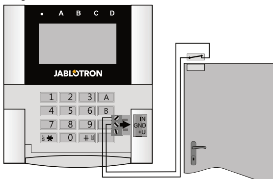
Figura 2: conexión de un contacto magnético
