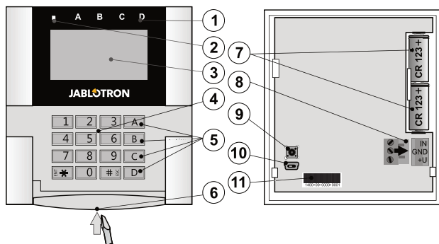
Figura 1: 1 – indicadores de estado A, B, C, D; 2 – indicador del sistema; 3 – pantalla LCD; 4 – teclado y lector RFID; 5 – botones de función A, B, C, D; 6 – pestaña para apertura de teclado; 7 – baterías; 8 – terminal BUS desmontable; 9 – contacto de sabotaje; 10 – conector mini USB; 11 – número de producción
