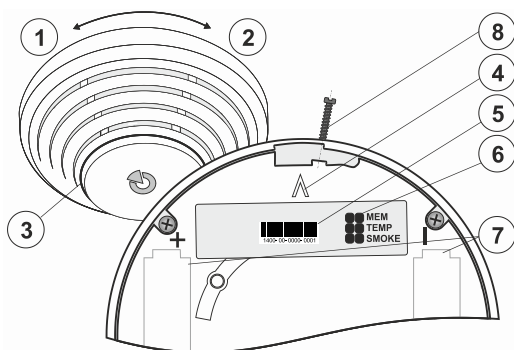
Afb. 6: 1 – het openen van het detectordeksel; 2 – het sluiten van het detectordeksel; 3 – signalering van de optische status; 4 – pijl, die aangeeft, waar de detector geplaatst dient te worden op het onderste deel; 5 – productiecode 6 – configuratiejumpers; 7 – batterijhouders; 8 – borgschroef.
