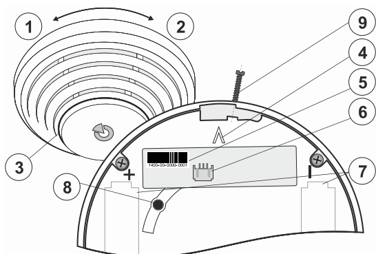
Fig. 6 : 1 - Ouverture du capot du détecteur ; 2 - Fermeture du capot du détecteur ; 3 - Signalisation optique d'état ; 4 - Flèche d'orientation pour le montage du détecteur ; 5 - Code de production ; 6 - Connecteur d'antenne externe ; 7 - Supports des piles ; 8 - Touche de test ; 9 - Vis d'arrêt
