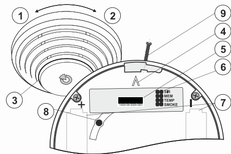
Fig. 6: 1 - detektordeksel åpnes; 2 - detektordeksel lukkes; 3 - varsling av optisk status; 4 - pil som viser hvor du skal sette inn detektoren; 5 - produksjonskode; 6 - konfigurasjonsterminaler; 7 - batteriholdere; 8 - knapp til testing 9 - festeskruer
