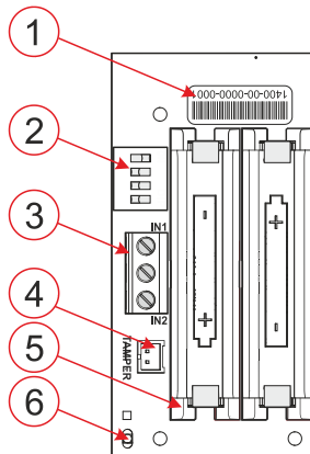
Obr. 1: 1 – sériové číslo, 2 – DIP prepínače pre nastavenie režimu vstupov, 3 – svorky vstupov IN1, IN2, C; 4 – konektor sabotážneho kontaktu, 5 – držiak batérií s vyznačenou polaritou, 6 – LED indikátor stavov;
