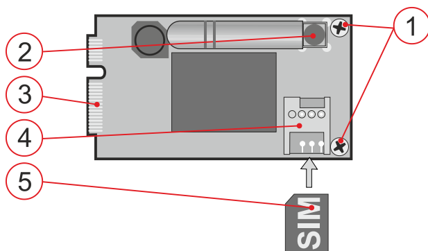
Figur 1: JA-194Y-kommunikationsmodul
