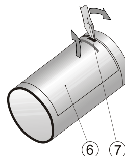
Afb. 3: 1 – indicator; 2 – batterijen; 3 – veiligheidsring; 6 – batterijdeksel; 7 – hulpgereedschap (een schroevendraaier);
