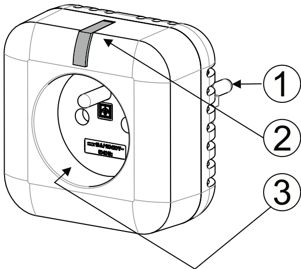
Obr. 1: 1 – vidlica typu UniSchuko; 2 – funkčné tlačidlo / kontrolka; 3 – zásuvka typ E – Francúzska zásuvka (French)
