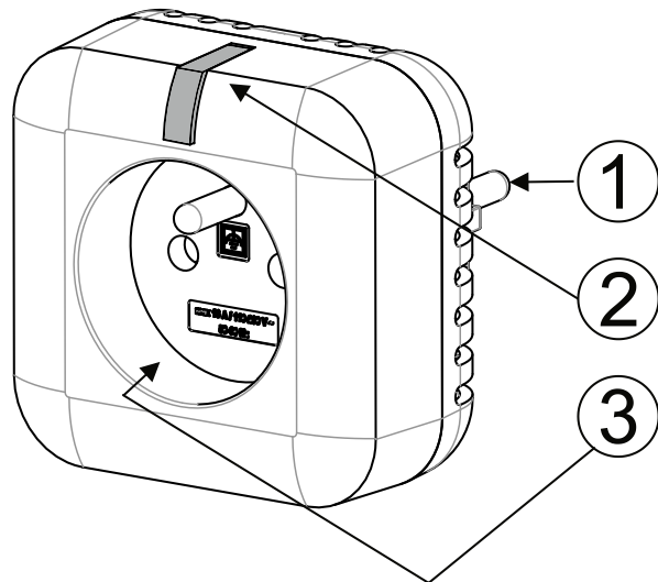
Fig. 1: 1 – UniSchuko-plugg; 2 – funktionsknapp / indikator; 3 – French-eluttag
